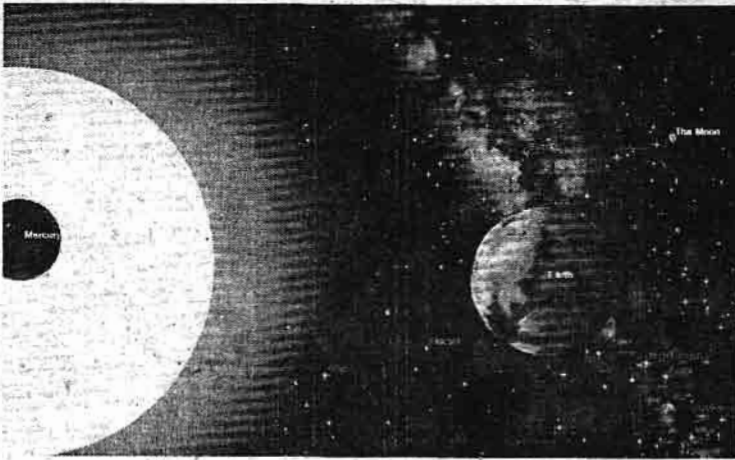
ဝဇ္ဇဟုဂြိုဟ် နေနှင့် ကမ္ဘာကြားထဲမှ လမင်းကြောင်းတည်မတ်စွာ ဖြတ်သန်းနေပုံ။
