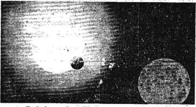
ကမ္ဘာဂြိုဟ်နှင့် နေနှင့် လကြားထဲသို့ လမ်းကြောင်းတည့်မတ်စွာ ရောက်ရှိပြီး လကြတ်သောဖြစ်စဉ် ဖြစ်ပေါ်လာပုံ
