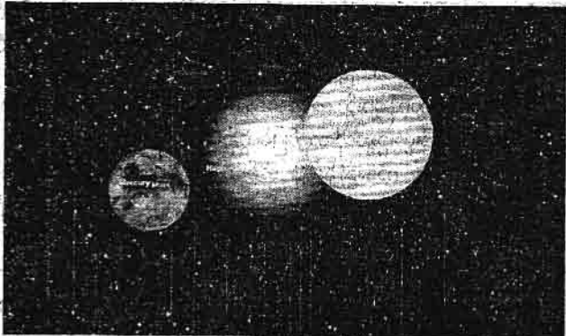
အင်္ဂါဂြိုဟ်နှင့် သောကြာဂြိုဟ်များ နေ၏ အနောက်ဘက် ဂြိုဟ်ပတ်လမ်းကြောင်းအတွင်း ပူးယှဉ်နေပုံ
