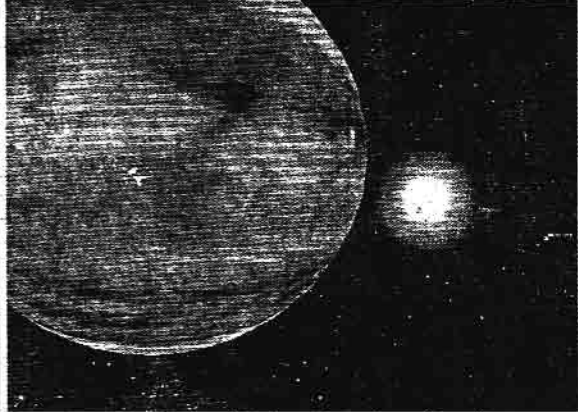
ကြာသပတေးဂြိုဟ်နေ့၏ အနောက်ဘက် ဂြိုဟ်ပတ်လမ်းကြောင်းထဲ ရောက်ရှိနေပုံ
