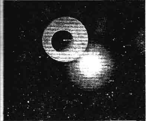
ဗုဒ္ဓဟူးနှင့် သောကြာဂြိုဟ်များ ပူးယှဉ်နေပုံ
