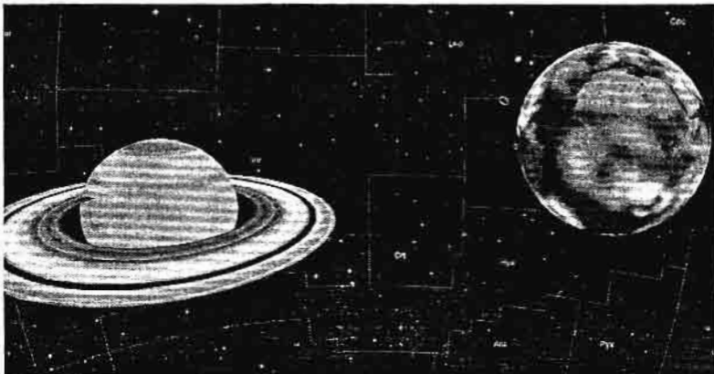
စနေဂြိုဟ် ကမ္ဘာ့ဘေးဘက် ဂြိုဟ်ပတ်လမ်းကြောင်းထဲ ရောက်ရှိပြီး ကမ္ဘာနှင့် တစ်တန်းတည်း ကျရောက်နေပုံ။
