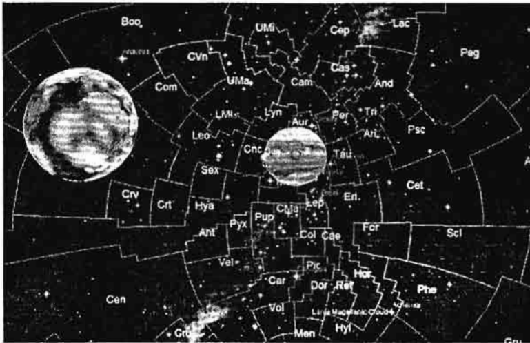
ကြာသပတေးနှင့် အင်္ဂါဂြိုဟ်များ ပူးယှဉ် စစ်ထိုးနေပုံ။
