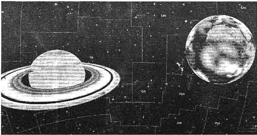
စနေဂြိုဟ် ကမ္ဘာနှင့် တစ်တန်းတည်း ကျရောက်နေပုံ။
