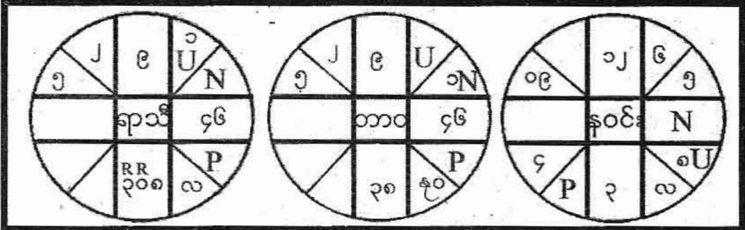
မလေးရှားနိုင်ငံ၊ ကွာလာလမ်ပူ လေဆိပ်မှ လေယာဉ် စတင်ထွက်ခွာချိန် ဇာတာခွင်၊
