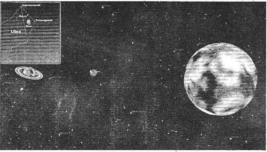
လနှင့် စနေဂြိုဟ်များ နီးကပ်စွာ ပူးယှဉ်နေပုံ။
