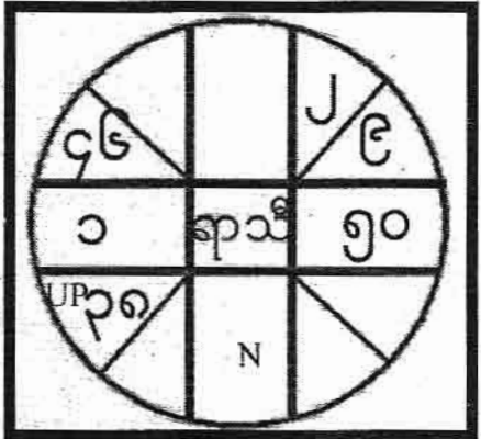
လေယာဉ်မှူး၏ ဇာတာခွင်
