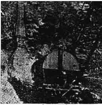
ယာယီရထားထမ်းမှ ရထားစက်ခေါင်းနှင့်တွဲများကို သံမဏိဆိုင်ကြီးများဖြင့် ဆွဲတင်၊ ဆွဲချ ပြုလုပ်ပေးနေသည့် မုတ်တမ်းအာတ်ပုံ
