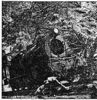
ဂုတ်တွင်း ခေါ်လျှိုကြီးအလယ်သို့ရောက်နေသော ရထားစက်ခေါင်းကြီးကို တစ်ဖက်ကမ်းသို့ သံမဏိဆိုင်ကြီးများဖြင့် ဆွဲတင်နေသည့် မုတ်တမ်းအာတ်ပုံ
