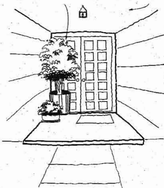
အသက်မွေးဝမ်းကျောင်းဆိုင်ရာ ကွာရှိရာ အိမ်ရှေ့တံခါးဝနေရာ၌ မထားရှိသင့်သောပုံစံများပြပုံ
