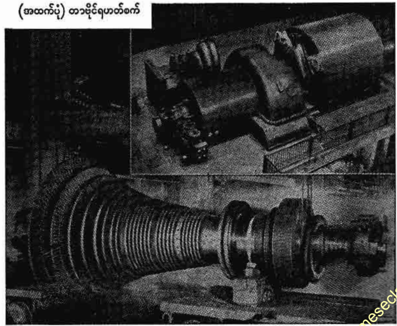
(အောက်ပုံ) ရေနှေးငွေ့ဖြင့်လည်သော တာဝိုင်ရဟတ်စက်၏ ဝင်ရိုးထံ
