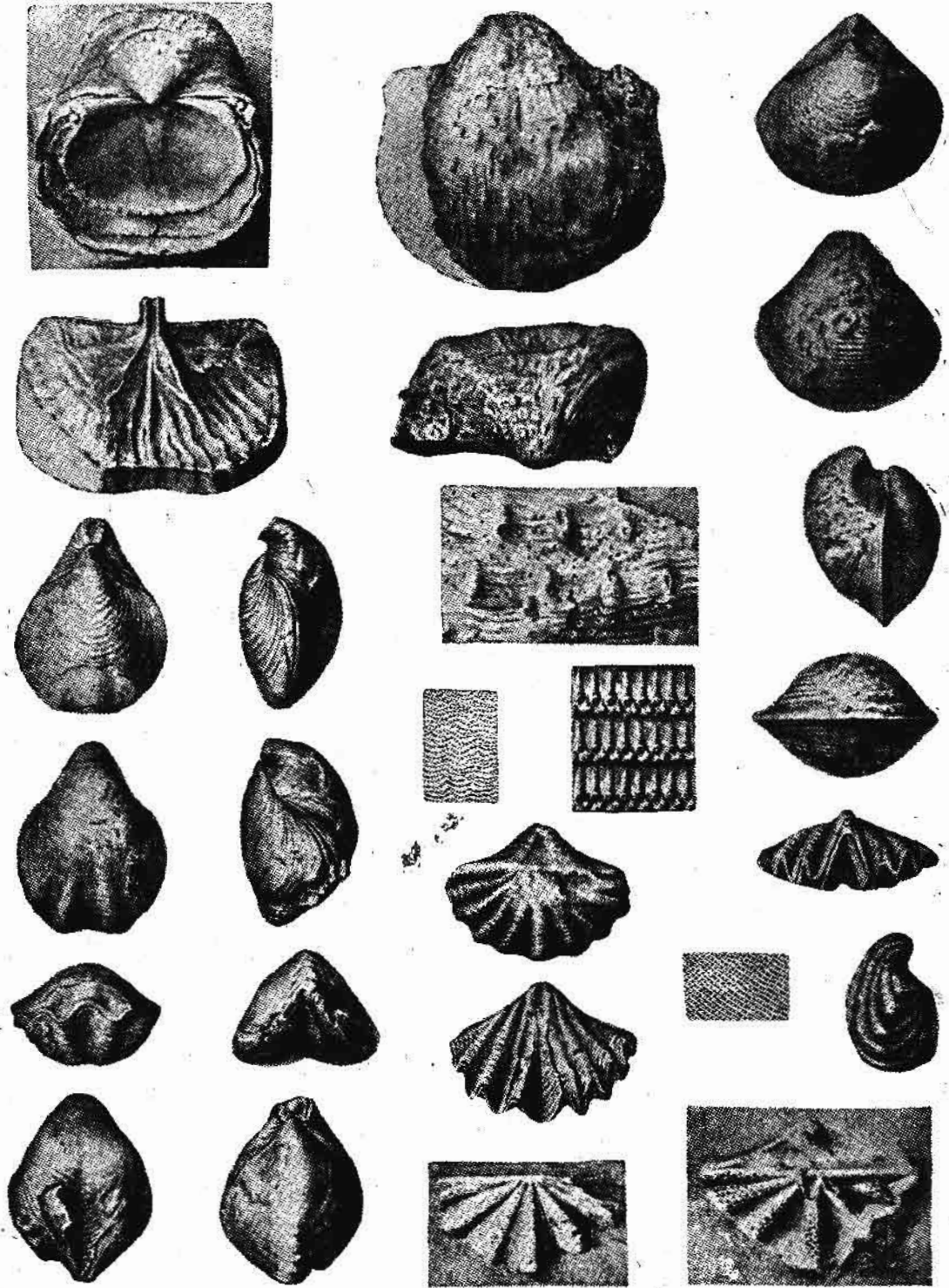
ထွန်ခဲ့သော နှစ်ပေါင်း သန်း ၃၀၀ ခန့်က ဖြစ်ပေါ်ခဲ့သော ရှမ်းပြည်တောင်ပိုင်းရှိ ကုန်းပြင်မြင့် ထုံးကျောက်လွှာများမှ ရရှိသော ရုပ်နှင်း ကျောက်များပုံဖြစ်သည်။ ယင်းကို လေ့လာသောပညာကို နိခါတက ဗေဒ ဟု ခေါ်သည်။
