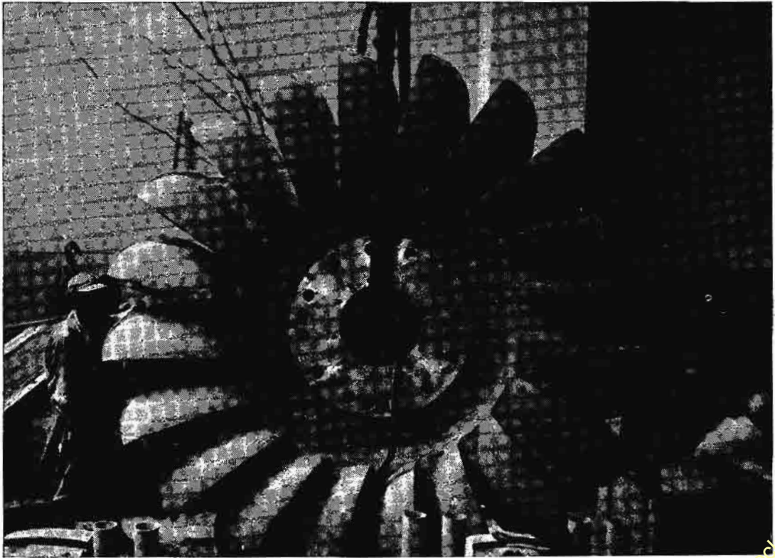
ရေအားမှ လျှပ်စစ်ဓာတ်အားအဖြစ်သို့ ပြောင်းလဲပေးမည့် ရေရဟတ်ကြီးတင် ခွက်ကြီးများ ပါရှိသည်။ ပန်းထွက်လာသော ရေအားသည် ထိုခွက်ကြီးများကိုအရှိန်ပြင်းစွာ တွန်းသဖြင့် ရဟတ်ကြီး လည်ရခြင်းဖြစ်သည်။
