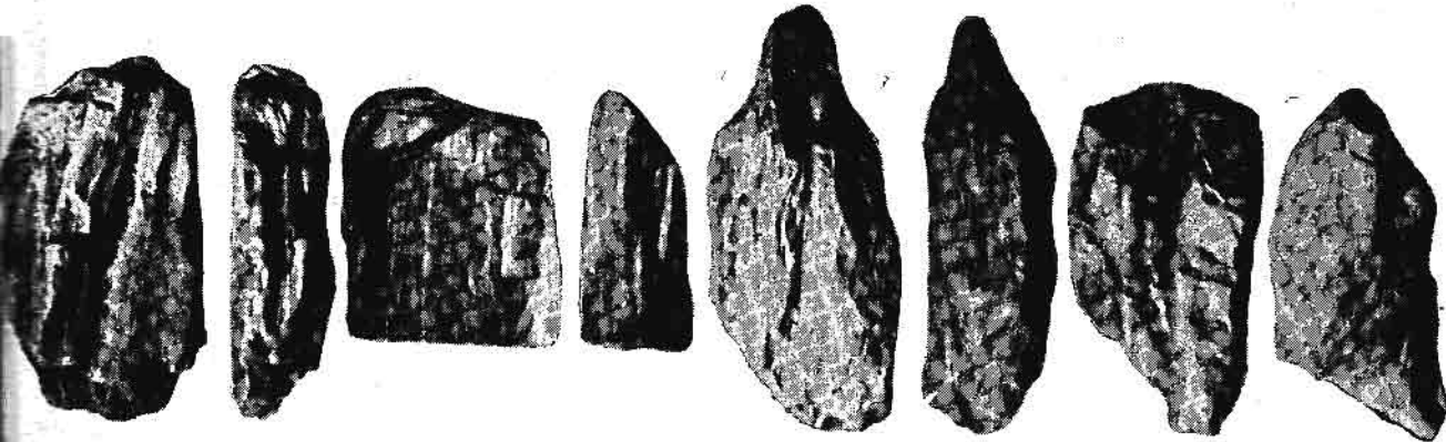
မြန်မာ့ကျောက်ခေတ်ဦးတွင် တွေ့ရှိရသော အင်ကြင်းကျောက်ဖြင့် ပြုလုပ်ထားသော လူသုံးကရိယာများ။ ညောင်ဦးမှ ရရှိသည်။
