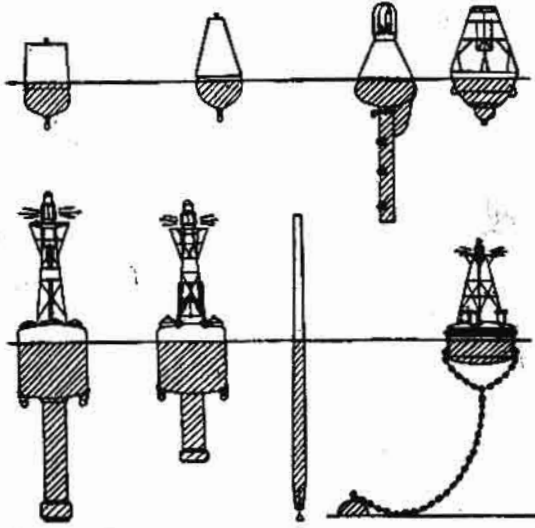
အပေါ် (ဝ) ရိုးရိုးဗော်ယာ ၂ မျိုးနှင့် (ယာ) ခေါင်းလောင်းတပ် အချက်ပေး ဗော်ယာ ၂ မျိုးတို့ဖြစ်ကြသည်။ အောက်ပုံများမှာမှ အပြေဗော်ယာများ ဖြစ်ကြသည်။
