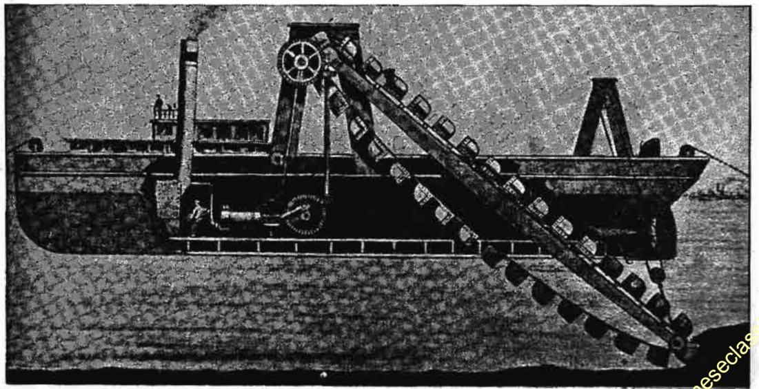
ခွံနှင့်သဲများကို ကျုံးယူနိုင်သောခွက်ကြီးများ ထပ်ဆင်ထားသည့် သောင်ဖျက်စက်
