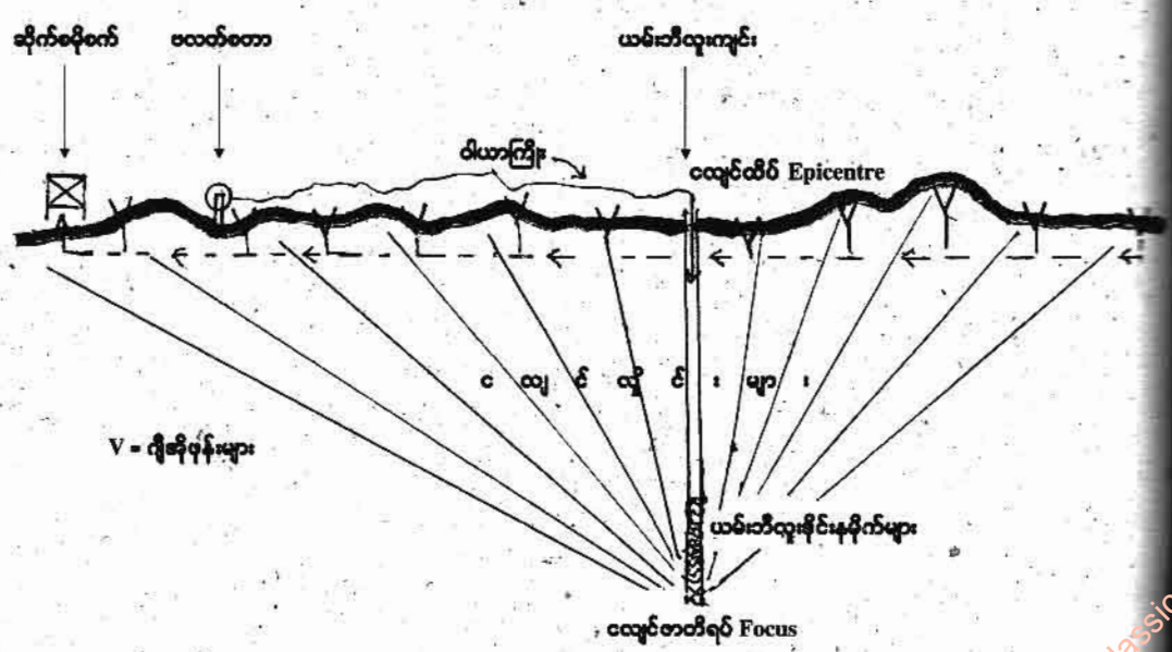
ဆိုက်စမစ်တိုင်းတာမှုသရုပ်ပြပုံကြမ်း
