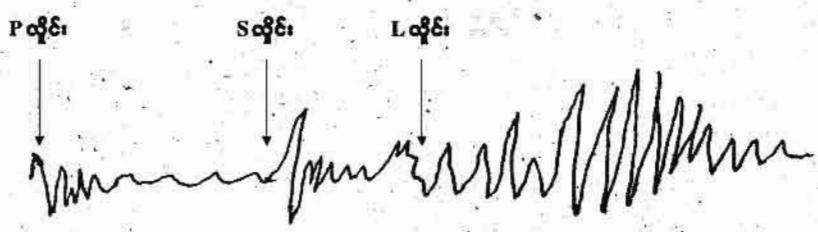
ဆိုက်စမစ်စက်မှ ဖလင်တွင် မြင်ရသော ငလျင်လှိုင်း
