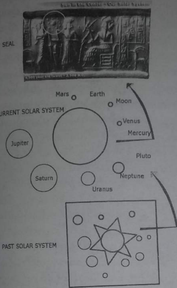
နေစကြဝဠာများနှိုင်းယှဉ်မှု
