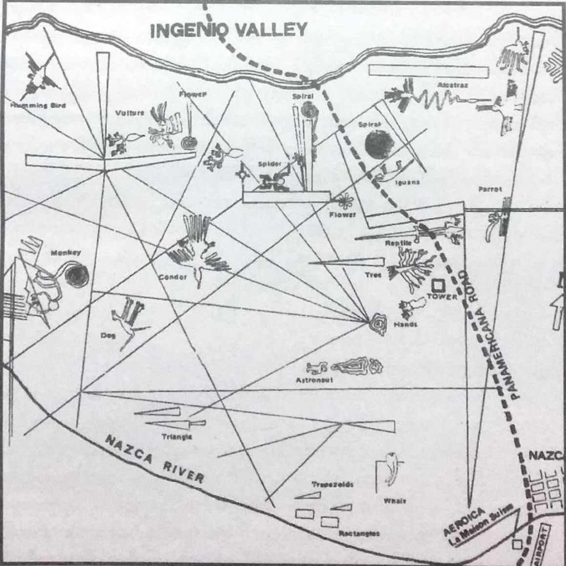
နက်ဖ်ကာ ဝေရီယာအတွင်း နက်ဖ်ကာလိုင်းများနှင့်ပုံများများဖြန့်ကျက်တည်ရှိနေပုံ
