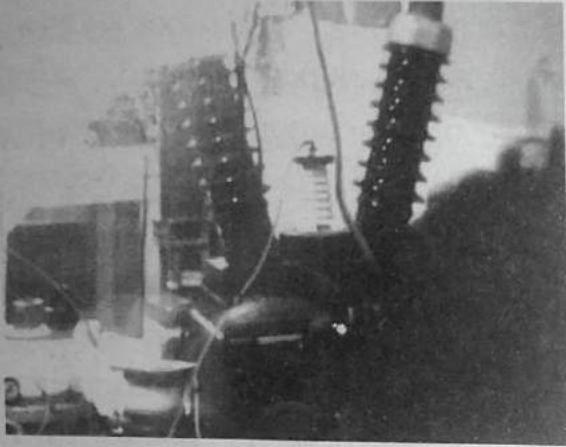
မြူခိုးများဖြစ်ထွန်းလာပုံ
