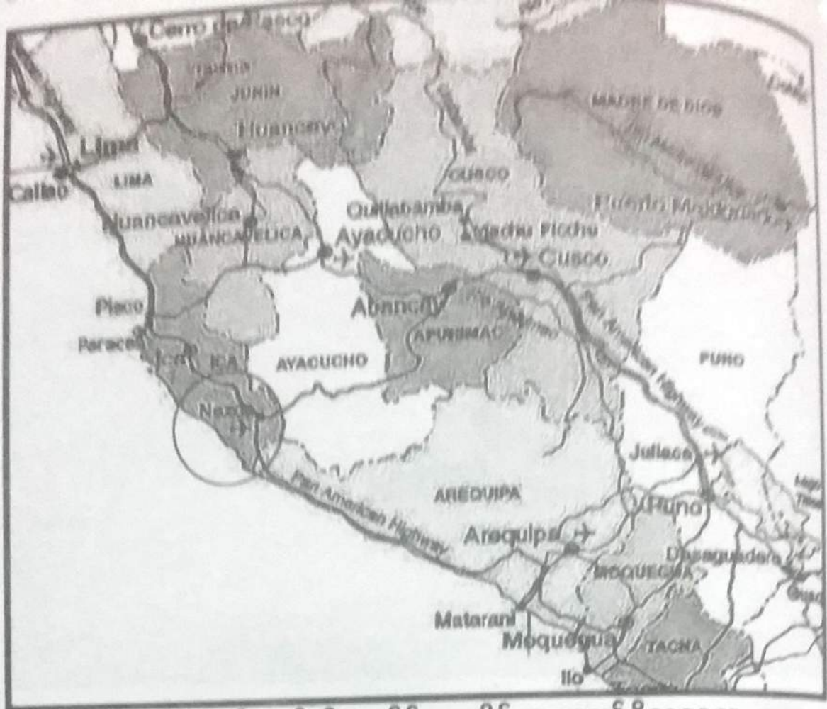
တောင်အမေရိကတိုက်၊ နက်စ်ကာလိုင်များတည်ရှိရာနေရာ
