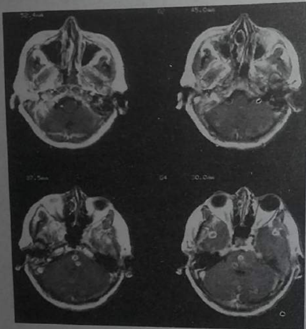
ဦးနှောက်အရွယ်အစားနှိုင်းယှဉ်ပုံ
