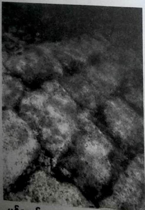
ပင်လယ်ရေအောက်မှတွေ့ရသော ဘီမိနီလမ်း
