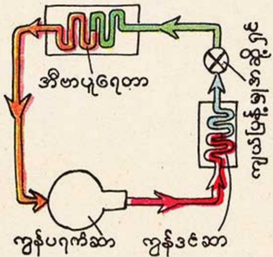
ဖိနှိပ်ခြင်း အမျိုးအစား အိမ်သုံးရေခဲသေတ္တာ အလုပ်လုပ်ပုံပြသောပုံစံ
