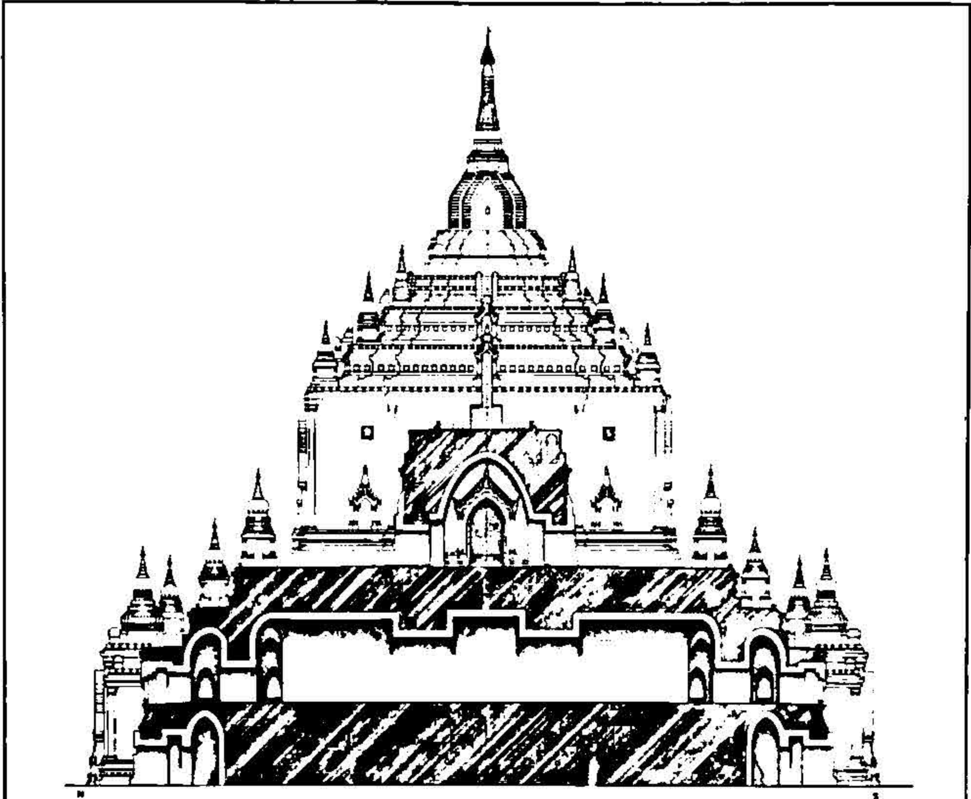
သဗ္ဗညုဘုရား တောင်-မြောက် ဖြတ်ပိုင်းပုံ
