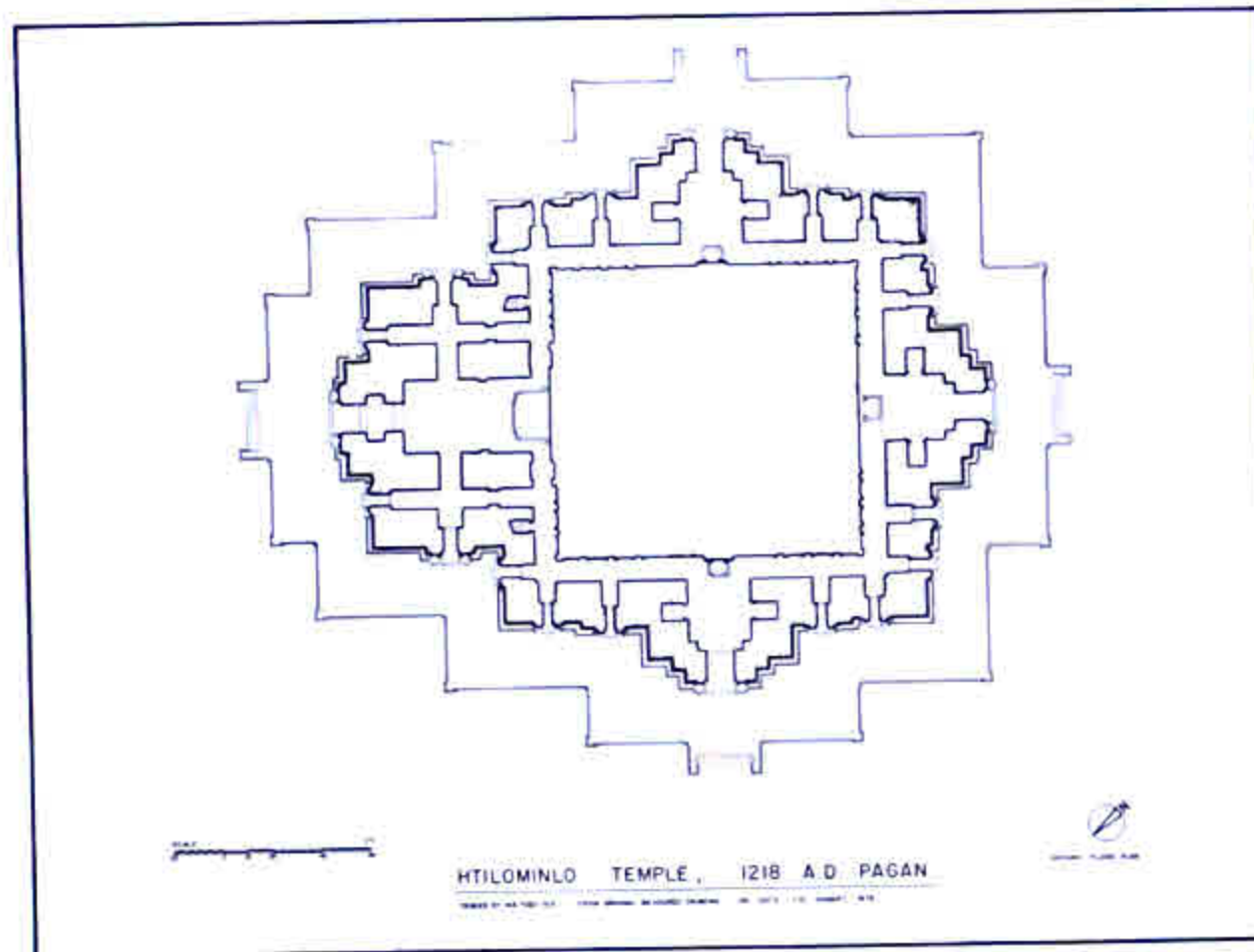
ထီးလိုမင်းလိုဘုရား မြေညီထပ် ပန္နက်ပုံ
