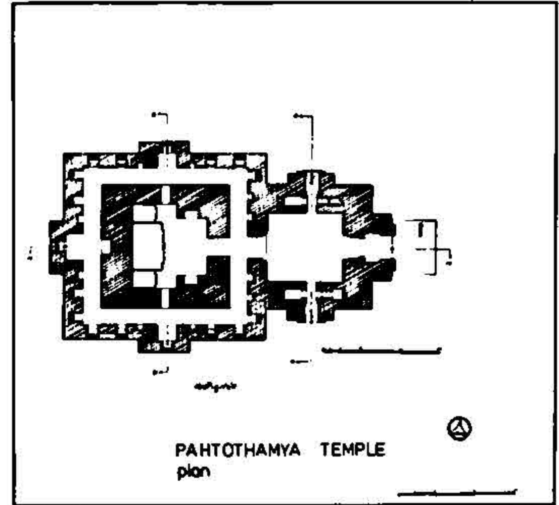
ပုထိုးသားများဘုရား ပန္နက်ပုံ
